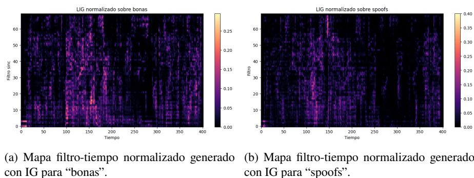
Figura 49: Mapas filtro-tiempo de la capa sinc-convolution generados con IG normalizados.
